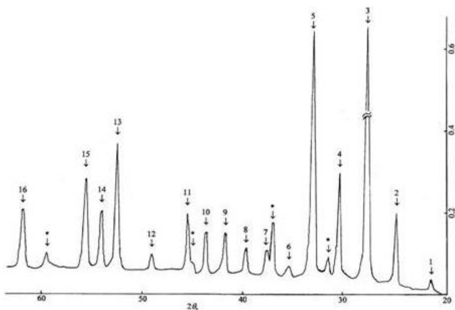
Fig. 5. Difrakția razelor X pentru produsul de piroliză a compusului declarat (cu puncte sunt indicate
